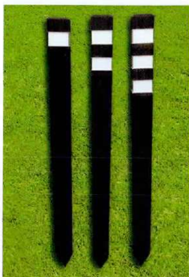
630-P 擬木ヤード杭角型 溝1本 擬木ヤード杭角型 溝2本 擬木ヤード杭角型 溝3本 70×70×1000mm 擬木製
